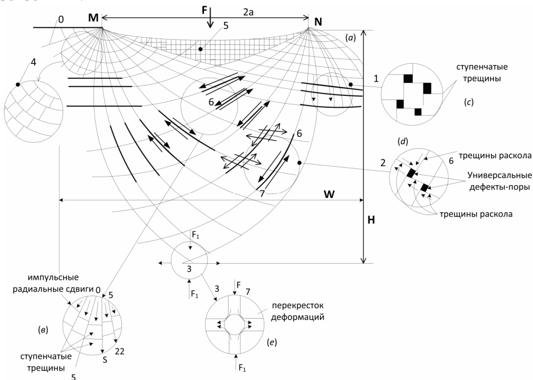
Рис. 3. Напряженное состояние в зоне деформации при внедрении шара (вертикальная сила). 5 – ЗЗД – зона затрудненной деформации; 0 – КТГ – коническая трещина Герца; W и H – ширина и глубина деформации; 1,2,3 – зоны образования трещин; 4 – образование ступеней и трещин на линиях сдвига: стрелочки – направление сил сдвига
