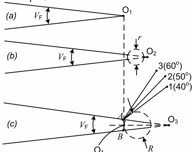
Рис. 1. Схема образования шарнира у ВУТ до создания разрушающего угла V_F : а) в хрупких материалах; б) квазихрупких материалах; в) пластичных, с образованием зоны вытяжки АВ и зоны предразрушений AO_3B
