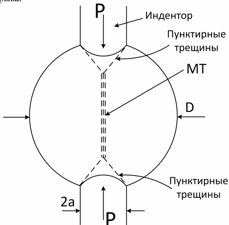
Рис. 4. Образец испытания по ASTM 2008, MT – магистральная трещина, D – диаметр образца, t – толщина образца
