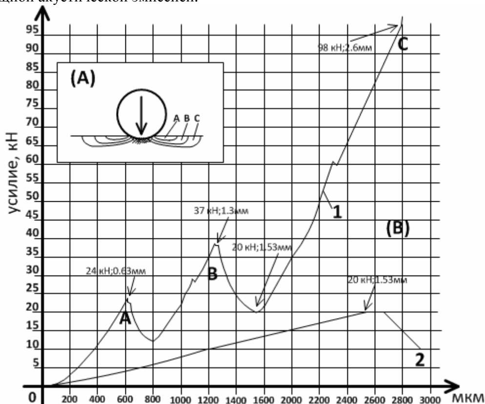
Рис. 2. Осциллограмма вдавливания шара диаметром 8 мм в гранит (в) – 1 и в органическое стекло (ПММА) – 2
